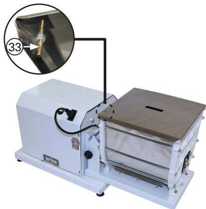
Misturador completamente montado
